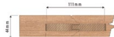
Dimension y posición de tarugos | Dowel dimension and position
